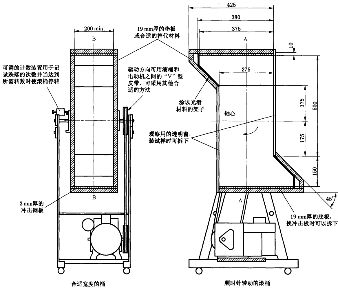
图 5 滚桶
