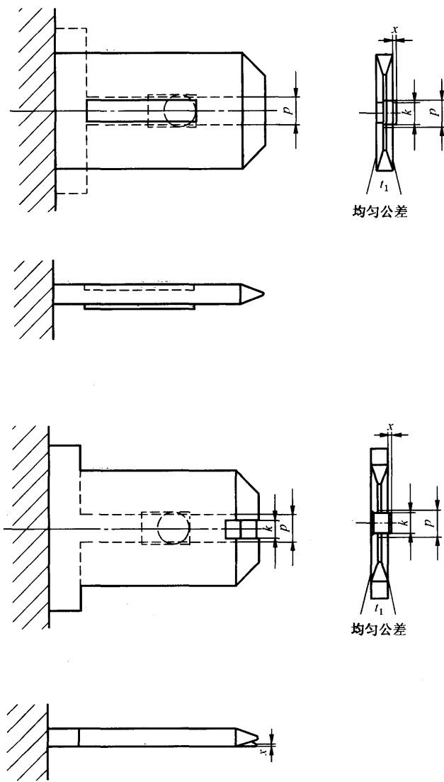
图 15 不可反接的连接器的插片
