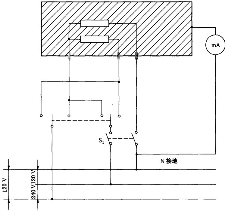
图 30 在工作温度下测量非Ⅱ类控制器在二相连接到三相中线接地电源上时泄漏电流的接线图
