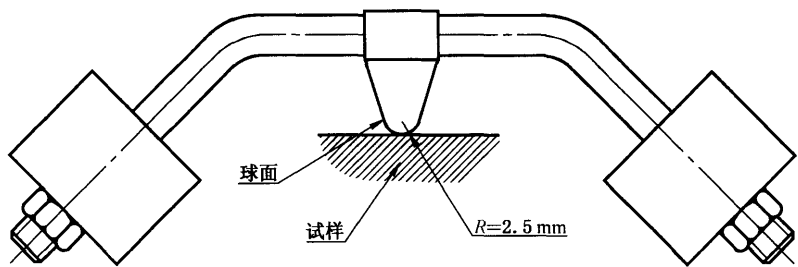
图 6 球压试验设备
