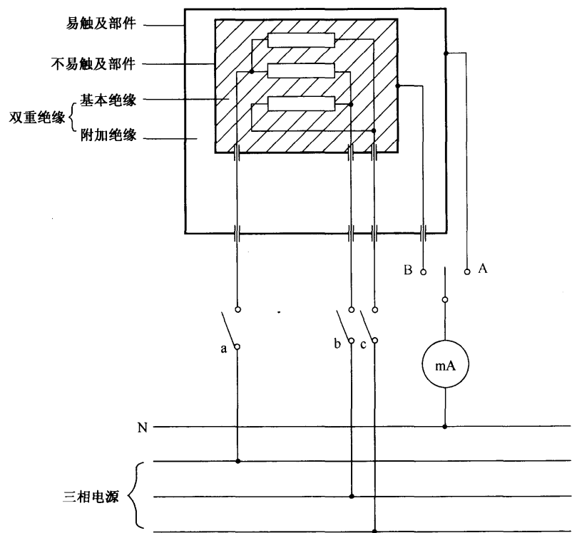
图 27 在工作温度下测量Ⅱ类控制器在三相连接时泄漏电流的接线图
