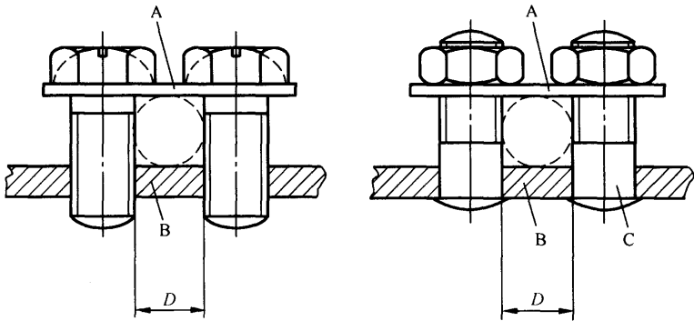
A——鞍架；B——固定部件；C——螺栓；D——导线所占空间图
