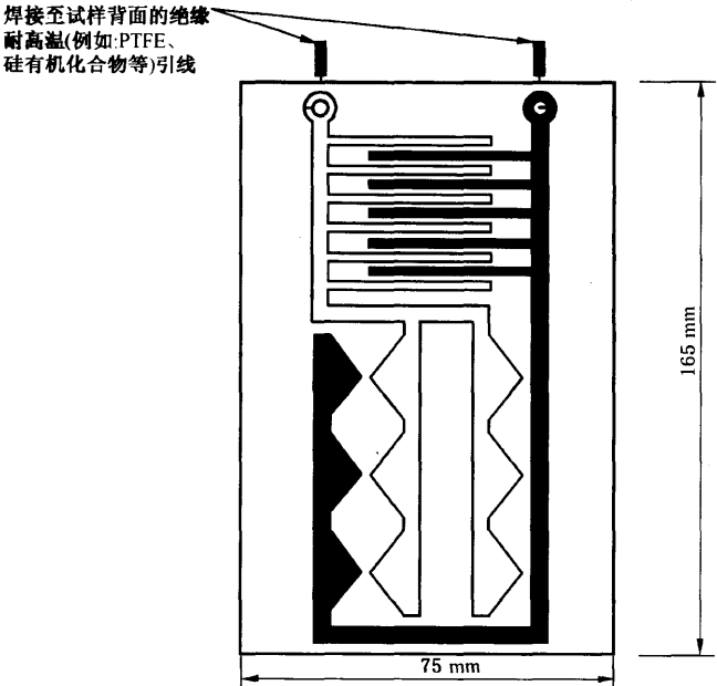
图 P.1 试验试样
