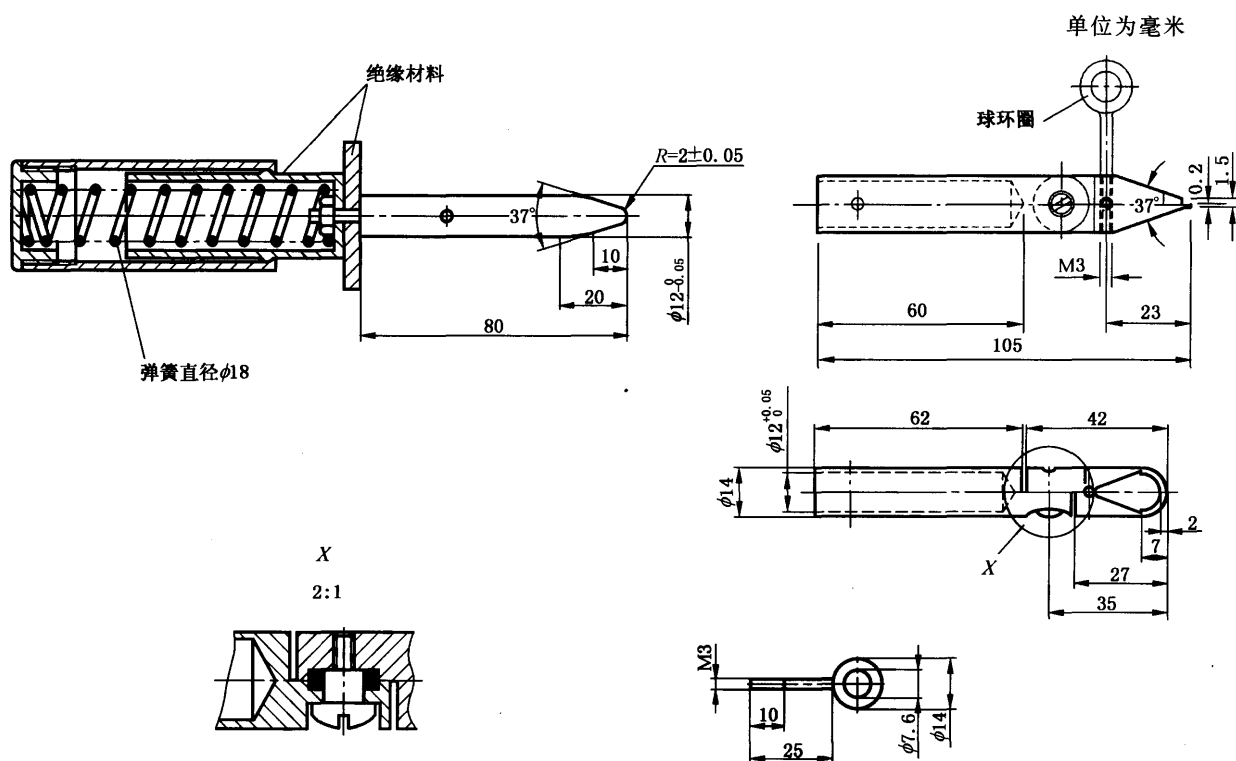
图 3 试验指甲
