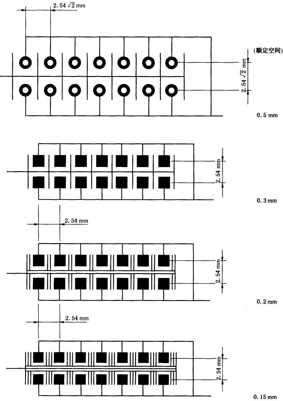
图 Q.2 焊盘分布图形示例(见图 Q.1)
