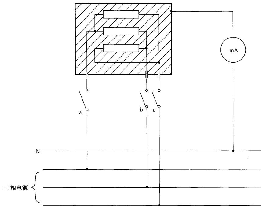
图 28 在工作温度下测量非Ⅱ类控制器在三相连接时泄漏电流的接线图
