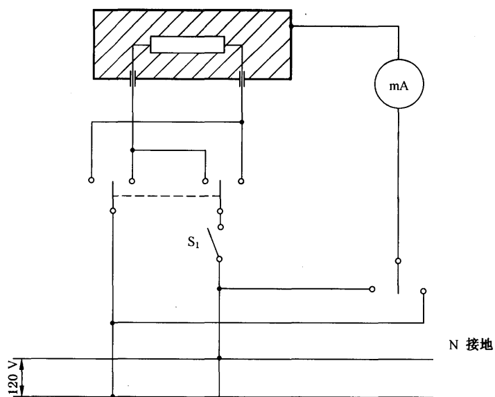
图 26 在工作温度下测量非Ⅱ类控制器在单相连接时泄漏电流的接线图
