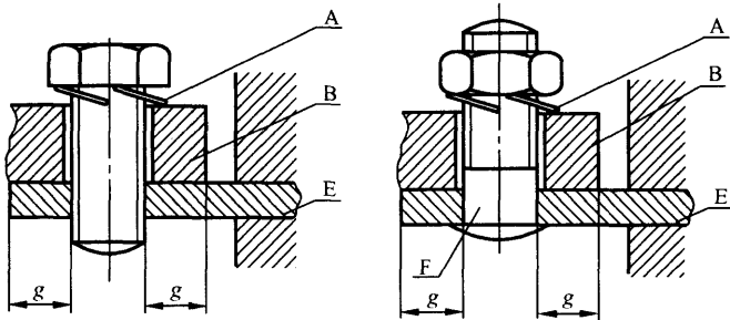
A——锁定措施；B——缆架或汇流条；E——固定部件；F——螺栓
