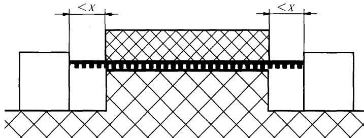
注：所考虑的路径包括一个未粘固的结合处以及一边一个宽度小于 X 的槽。 规则：爬电距离路径和间隙路径都是“视线”路径。
