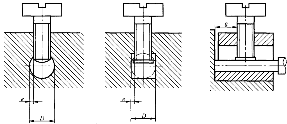
不带夹紧板的端子
