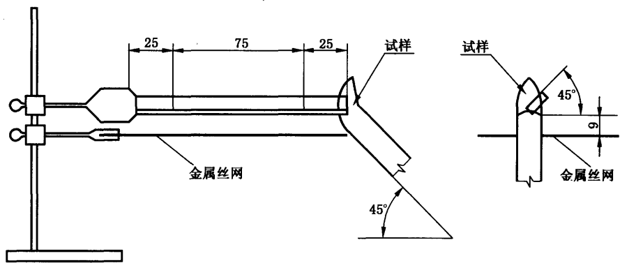
图 7 水平燃烧试验
