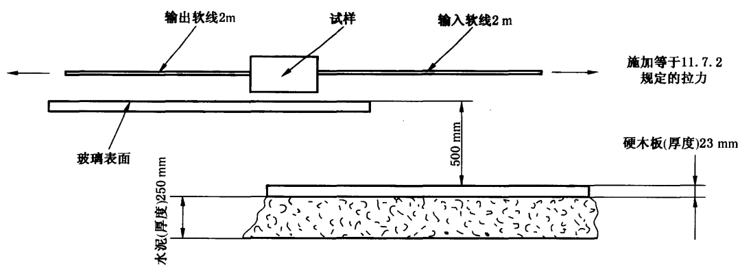
图 4 立式控制器的冲击试验
