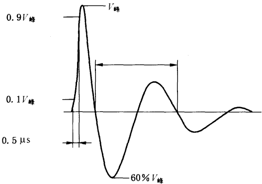
图 H. 26. 10. 1 振铃波特性(开路电压)
