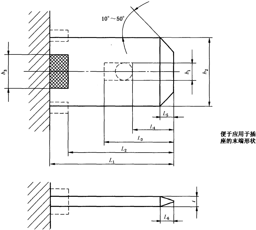
图 14 插片
