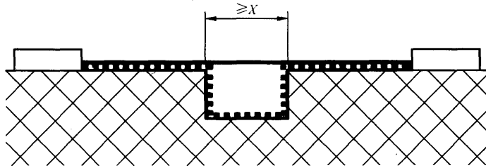
注：所考虑的路径包括宽度等于或大于 X 的槽。 规则：间隙路径是“视线”路径。 爬电距离是沿槽的轮廓路径。
