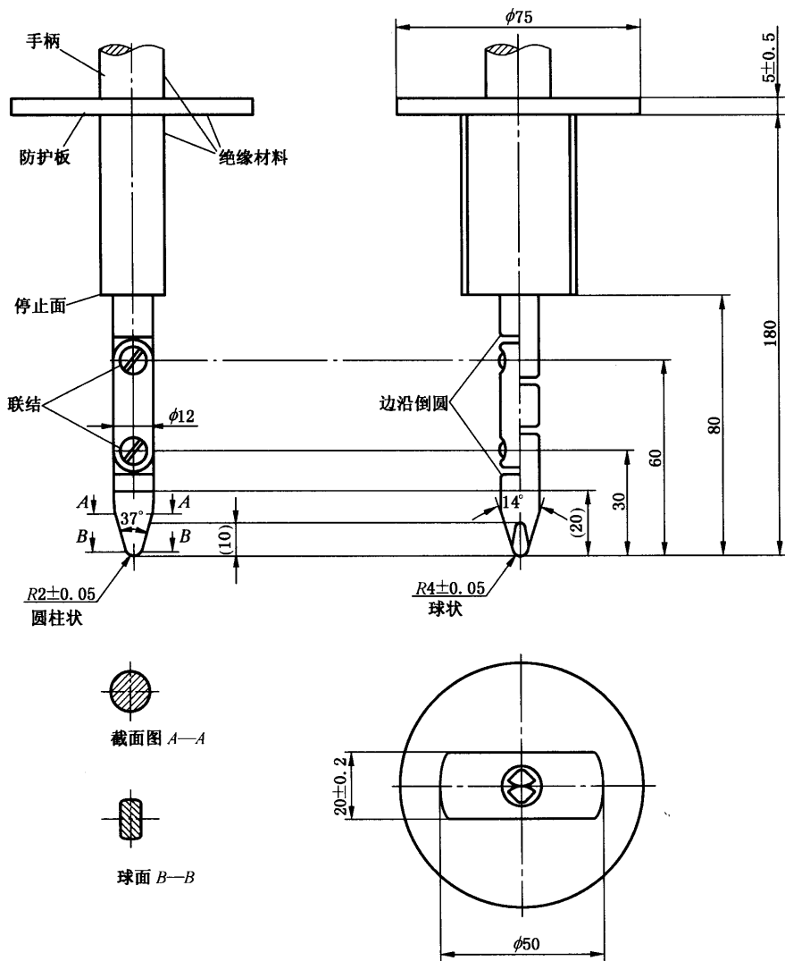
图 1 试验针
