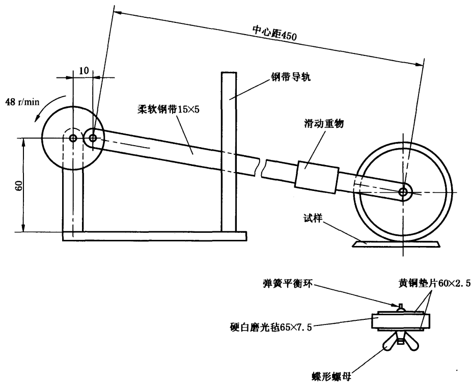
图 8 试验标签耐久性的设备
