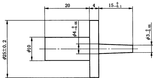
图 1 试验针
