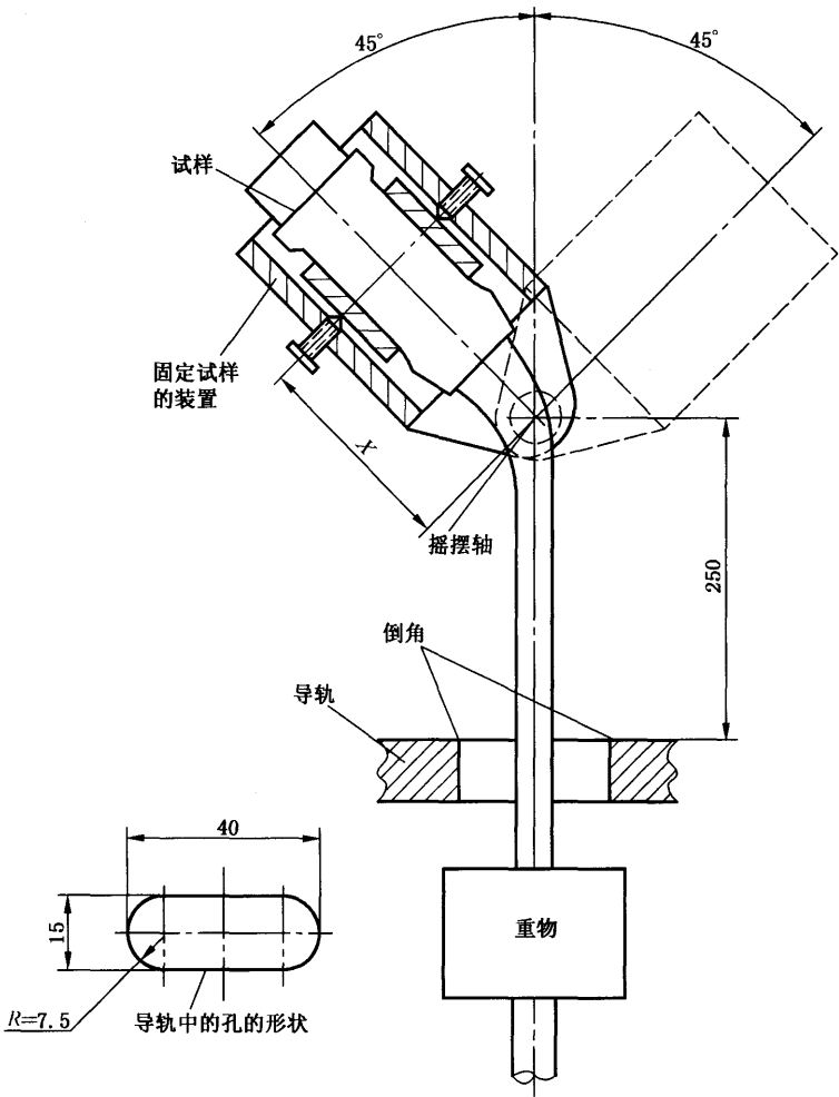
图 9 弯曲试验设备
