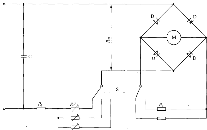
图 E.1 测量泄漏电流的电路
