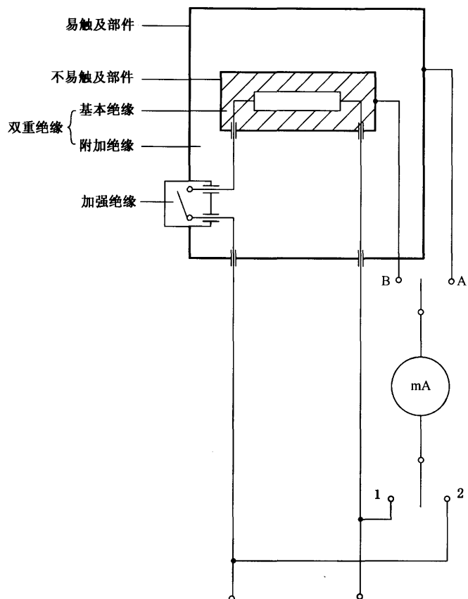
图 25 在工作温度下测量Ⅱ类控制器在单相连接时泄漏电流的接线图
