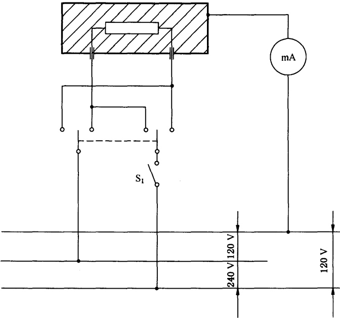
图 29 在工作温度下测量非Ⅱ类控制器在单相连接时泄漏电流的接线图
