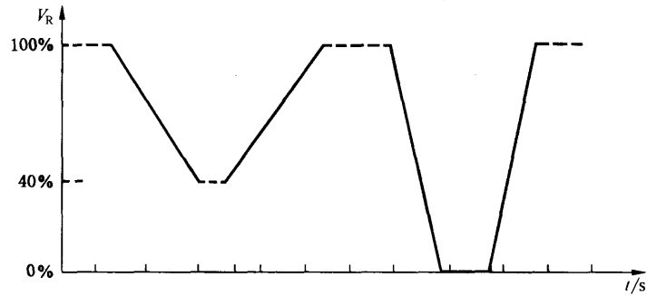
图 H. 26.5.4.2 电压变化测试
