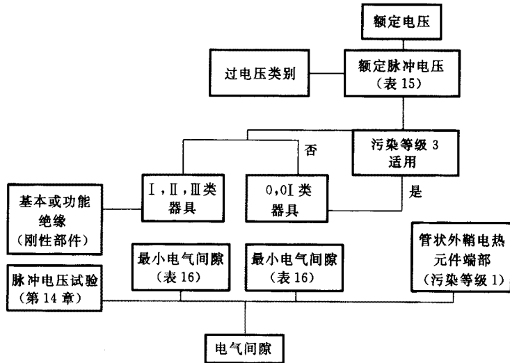
图 L.1 测定电气间隙的程序
